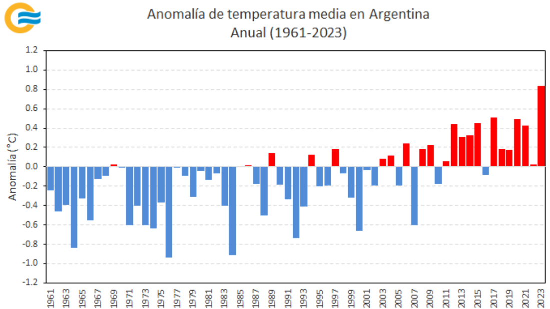
Figura 2.1. Anomalías de temperatura media en Argentina desde 1961 a 2023, con respecto al valor medio 1991-2020. En barras rojas se representan las anomalías positivas y en barras azules, las negativas.
