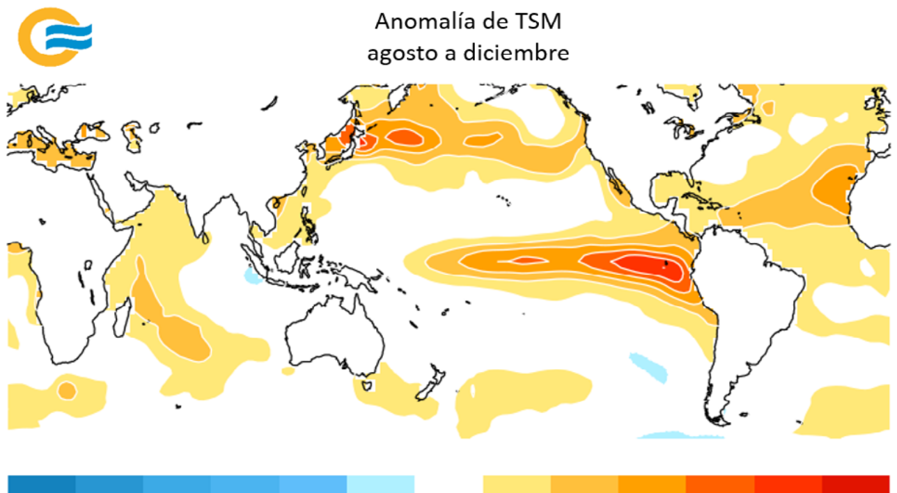
Figura 3.1. Promedio de anomalía de TSM entre el 1 de agosto y el 31 de diciembre de 2023. Fuente de datos: NOAA/ESRL. Graficado por el SMN.
