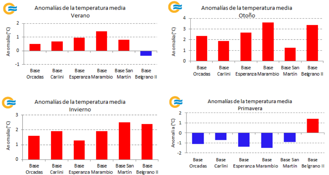
Figura 2.24. Anomalías de temperatura media de verano (arriba izq.), otoño (arriba der.), invierno (abajo der.) y primavera (abajo der.) para las bases Orcadas, Carlini, Esperanza, Marambio, San Martín y Belgrano II durante 2023, con respecto al valor medio 1991-2020. En barras rojas se representan las anomalías positivas y en barras azules, las negativas.
