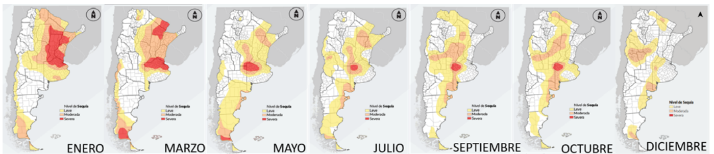
Figura 2.18. Evolución de las regiones de sequía durante 2023, de acuerdo a la Mesa Nacional de Monitoreo de Sequías. Fuente: https://www.magyp.gob.ar/sitio/areas/d_edu/sequia/
